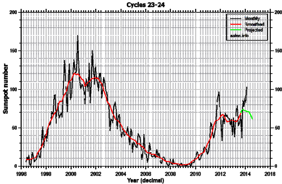
Bild 1: Sonnenzyklen 23 und 24. Quelle: www.solen.info
