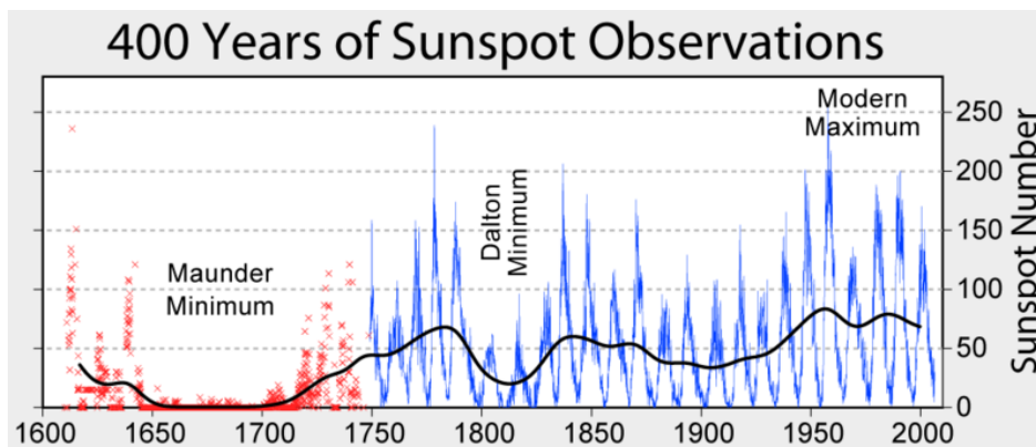
Bild 2: Sonnenflecken in den letzten 400 Jahren. Quelle: www.wikipedia.org
